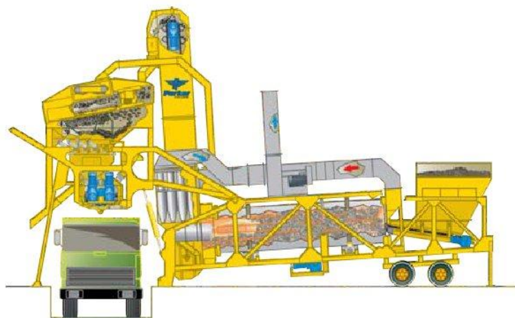
Option 1: Завод «Super-Roadmix» с комбинированной секцией загрузки из 2 бункеров
