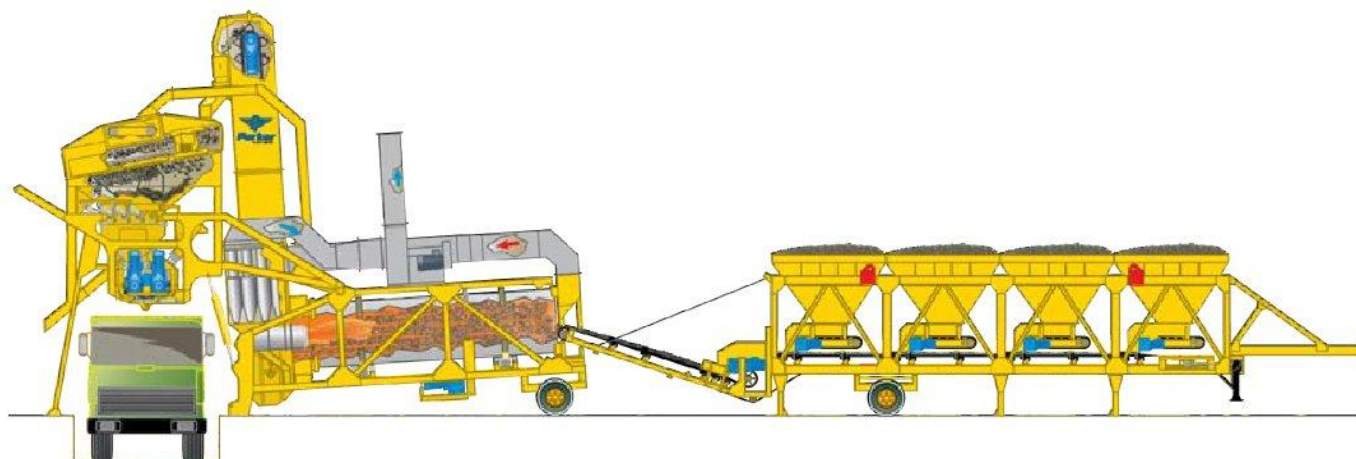
Option 2:* Завод «Super-RoadMix» с отдельной секцией загрузки из 3 или 4 бункеров
